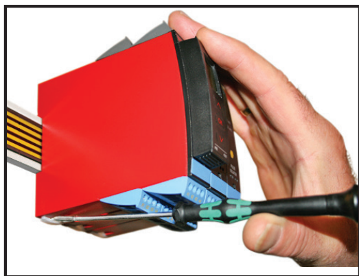
Figura 1: Levantando o botão de trava, o equipamento é destacado do trilho DIN.
